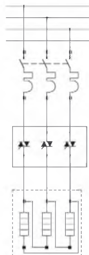
Трехфазное ТТР SCT/SVT/SGT для управления нагревательными элементами, соединенными треугольником, с автоматическим выключателем
