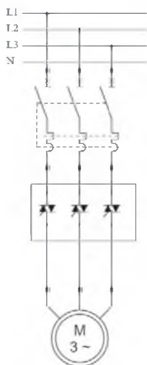
Трехфазное ТТР SVT8/SGT8, управляющее трехфазным двигателем, с термомангнитной защитой
