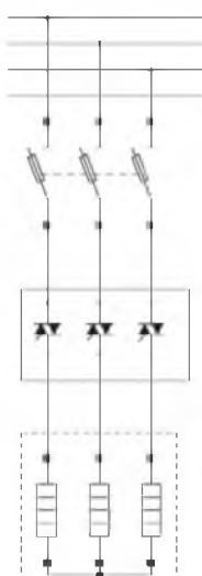
Трехфазное ТТР SCT/SVT/SGT для управления нагревательными элементами, соединенными звездой, с предохранителями
