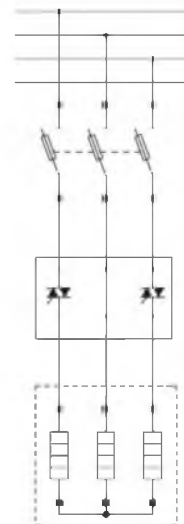
Двухконтактное трехфазное ТТР SGB для управления нагревательными элементами, соединенными звездой, с предохранителями
